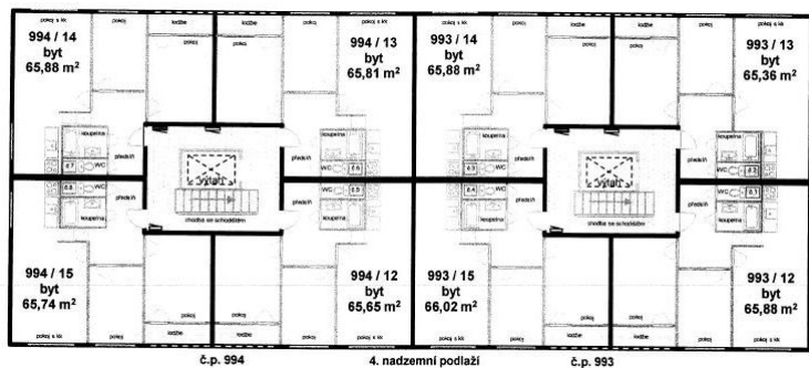
4. nadzemní podlaží
