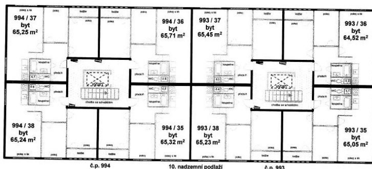
10. nadzemní podlaží
