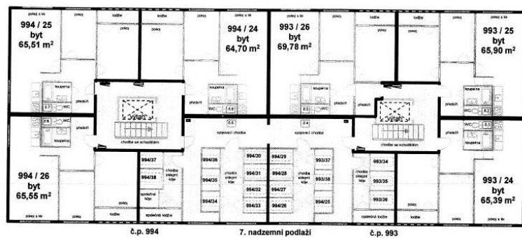
7. nadzemní podlaží
