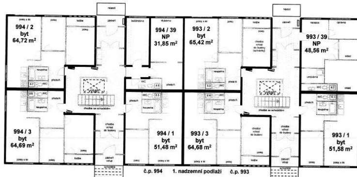
1. nadzemní podlaží
